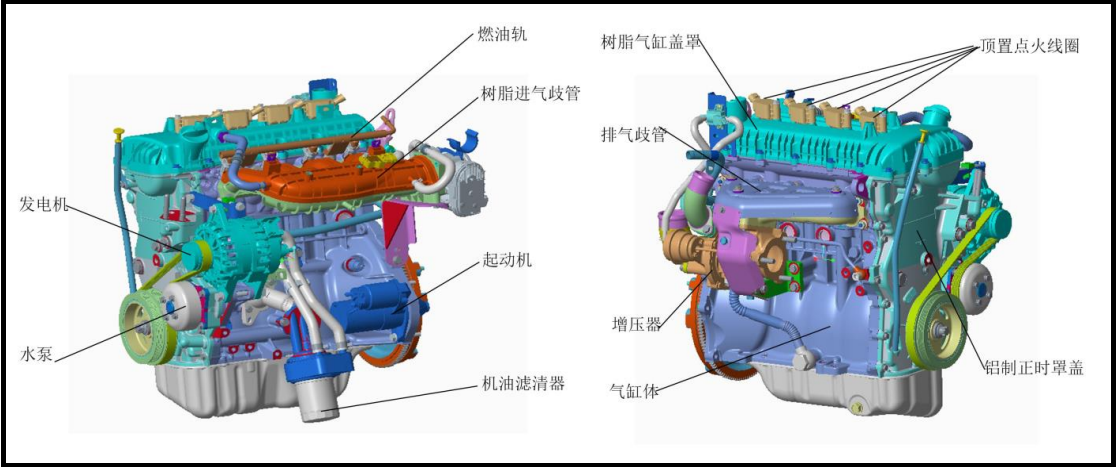
JT15T 发动机外观图：
